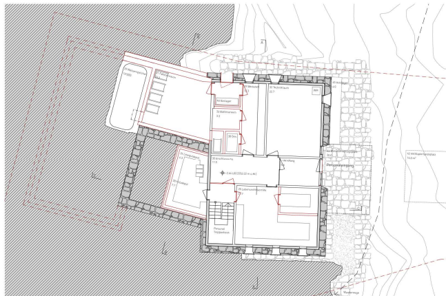
-1. Untergeschoss 1:100
