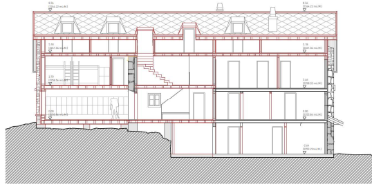
Längsschnitt C-C 1:100
