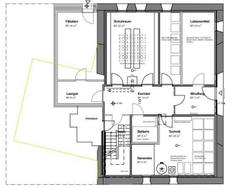
Untergeschoss 1/100
