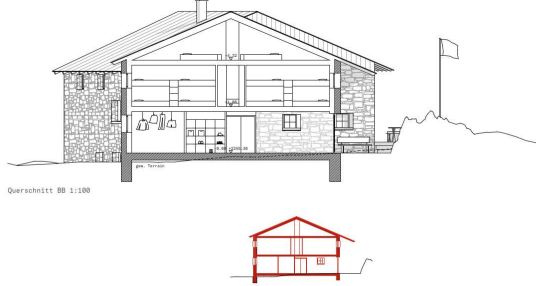
Abbruch/Neubau 1:250
