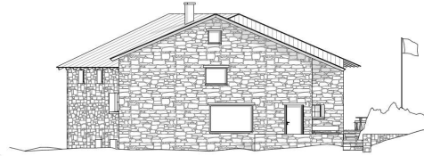
Westfassade 1:100
