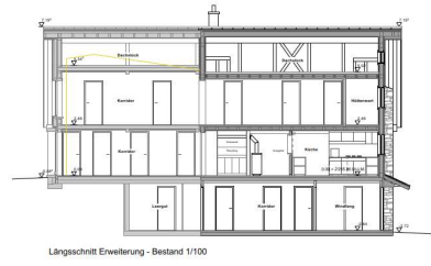
Längsschnitt Erweiterung - Bestand 1/100
