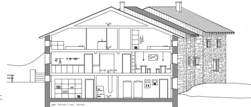
Querschnitt AA 1:100
