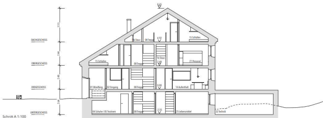
Schnitt A 1:100
