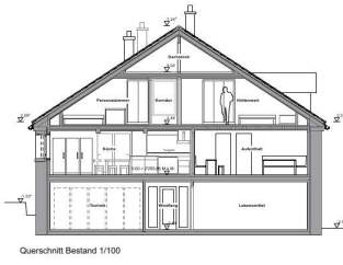
Querschnitt Bestand 1/100
