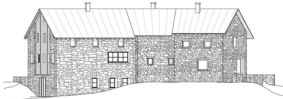
Nordfassade 1:100
