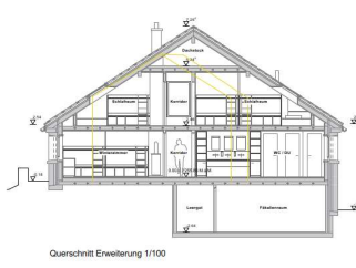
Querschnitt Erweiterung 1/100
