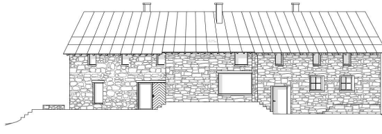
Südfassade 1:100
