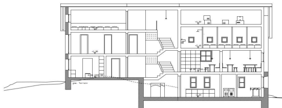
Längsschnitt CC 1:100
