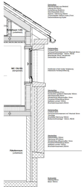
Fassadenschnitt Anbau/100
