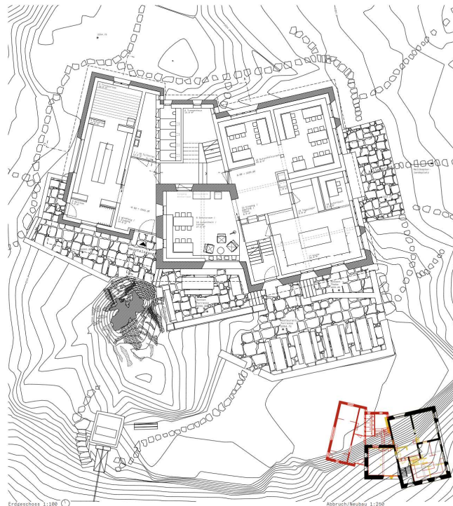
Erdgeschoss 1:100
