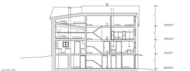
Schnitt B 1:100
