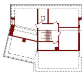
Abbruch-Neu Dachgeschoss 1:200
