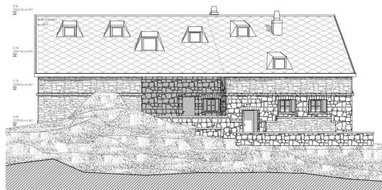
Ansicht Süden 1:100
