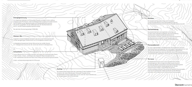
Übersicht isometrisch
